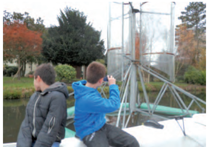
Une hydrolienne
